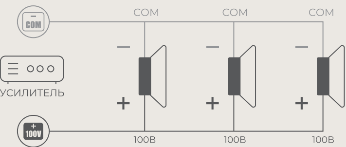
Параллельное соединение громкоговорителей
