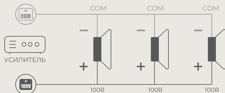
Параллельное соединение громкоговорителей
